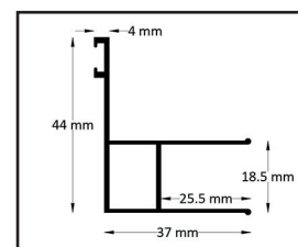
Profil zamykający drzwi
