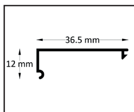
Pokrywa profilu przyściennego
