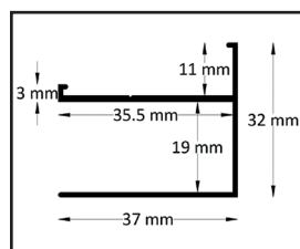
Profil przyścienny
