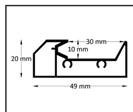
Profil prowadnicy
