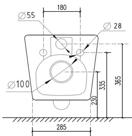
CUVETTE (art.GIO.24RIM)
