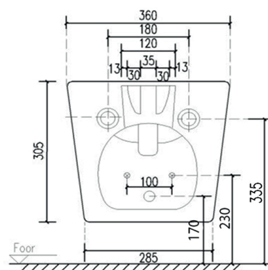
BIDET (art.GIO.25RIM)
