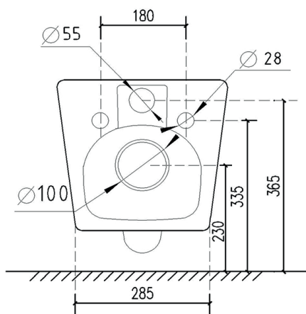
VASO (art.GIO.24RIM)
