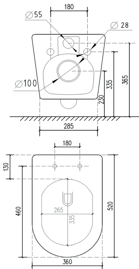
WC (art.GIO.24RIM)
