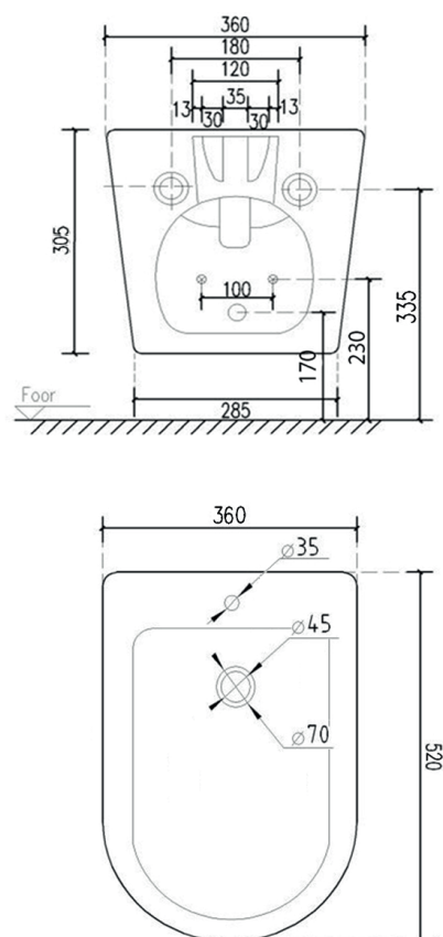
BIDET (art.GIO.25RIM)
