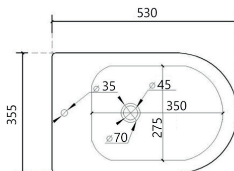
BIDÉ (art.GIO.27RIM)
