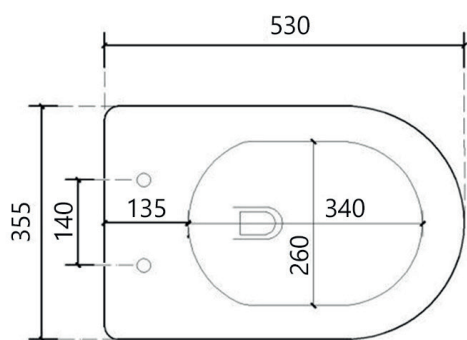
INODORO (art.GIO.26RIM)
