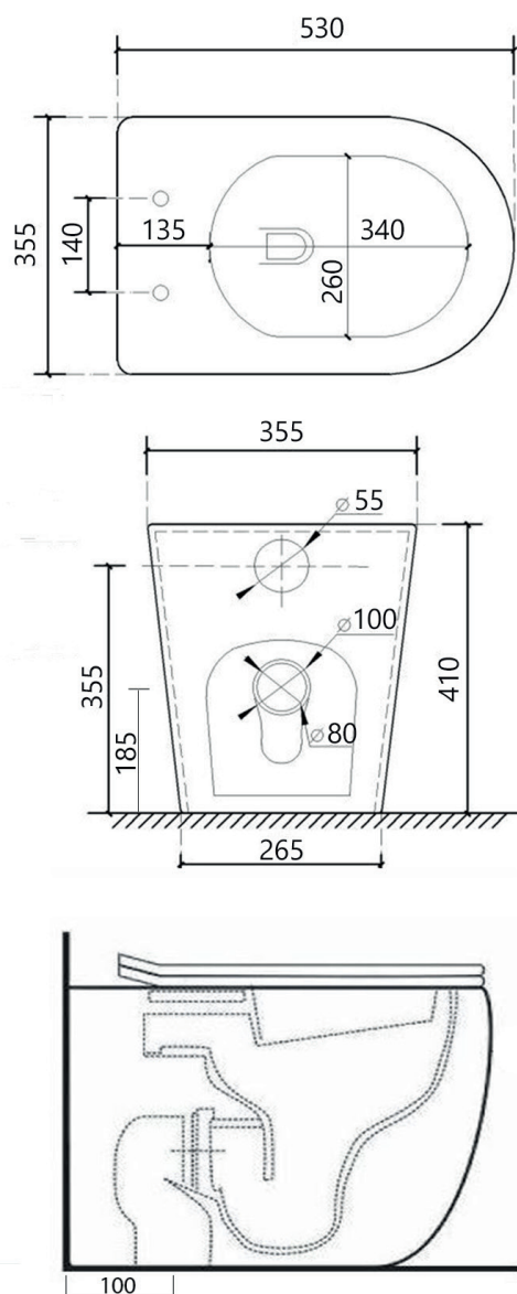
CUVETTE (art.GIO.26RIM)
