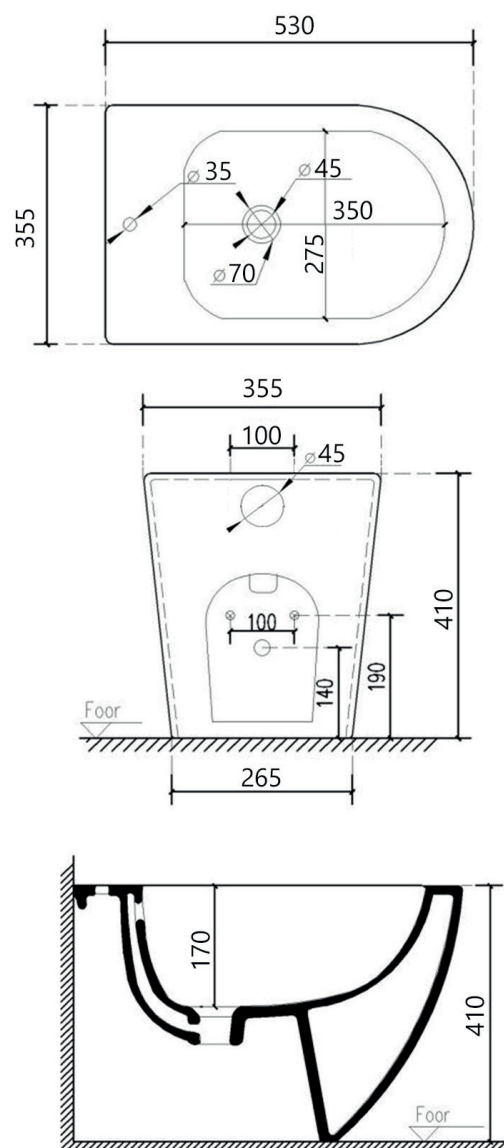
BIDET (art.GIO.27RIM)
