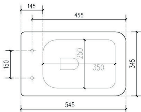
INODORO (art.GIO.22RIM)
