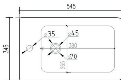
BIDÉ (art.GIO.23RIM)
