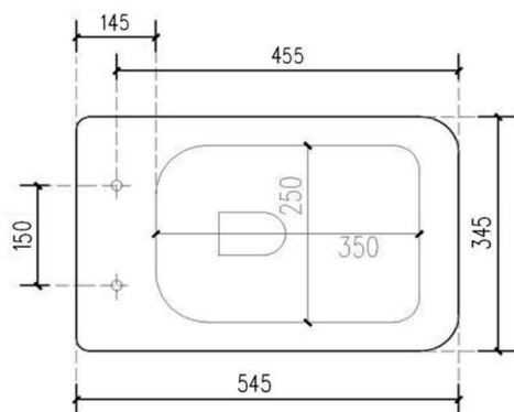
CUVETTE (art.GIO.22RIM)
