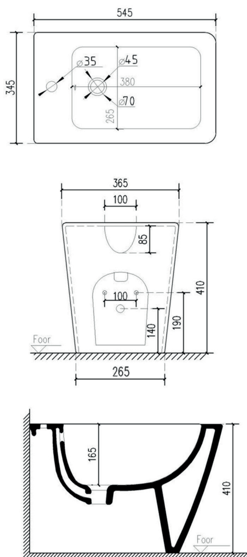
BIDET (art.GIO.23RIM)
