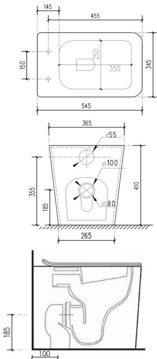
TOILET (art.GIO.22RIM)
