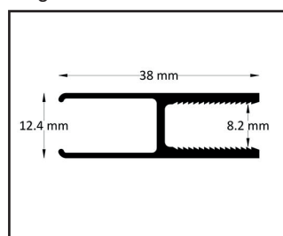
Festes Glasprofil
