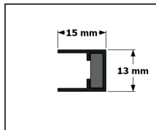
Magnet-Profil
