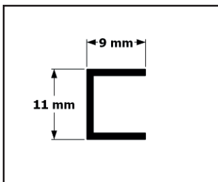
Schließendes Seitenwandprofil
