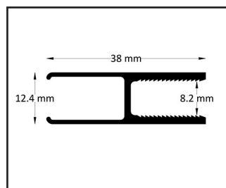
Profilé de verre fixe
