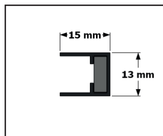
Profil de l'aimant
