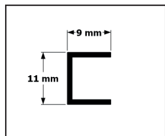
Profil przyścienny strony zamknięcia
