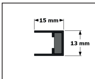
Profil magnetyczny
