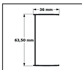
Wandprofil
