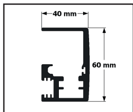
Perfil carril
