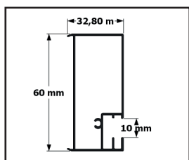
Perfil de cristal fijo
