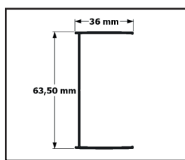
Perfil de la pared
