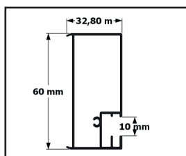
Profil szkła stałego
