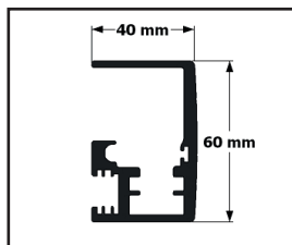
Profil prowadniczy
