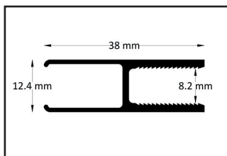
Glasprofil
