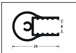
Drehbares Scharnierprofil
