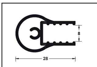
Perfil de bisagra giratoria
