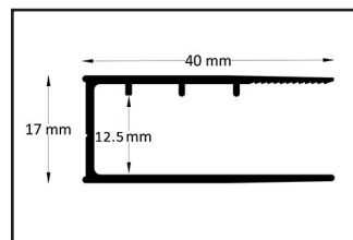
Perfil de la pared
