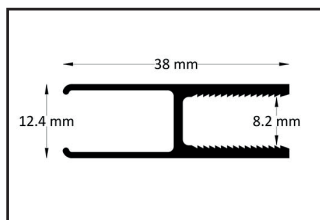
profilé verre
