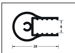
Profilo cerniera rotante
