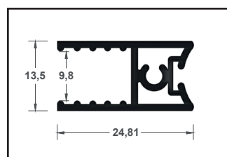
Profilo cerniera fissa
