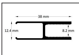
Profilo vetro
