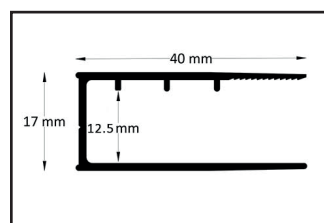
Profilo muro
