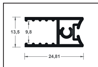
Profil zawiasu stałego
