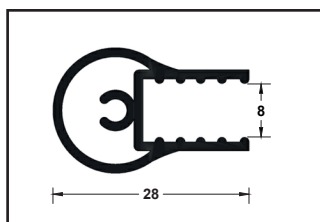
Profil zawiasu obrotowego
