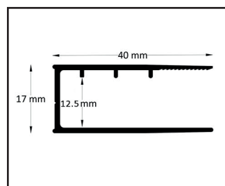
Profil wall
