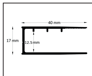
Profilo muro
