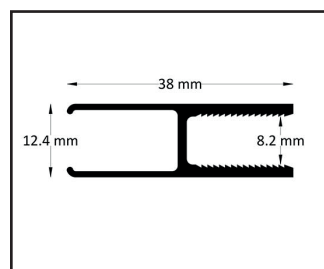
Profil szkła
